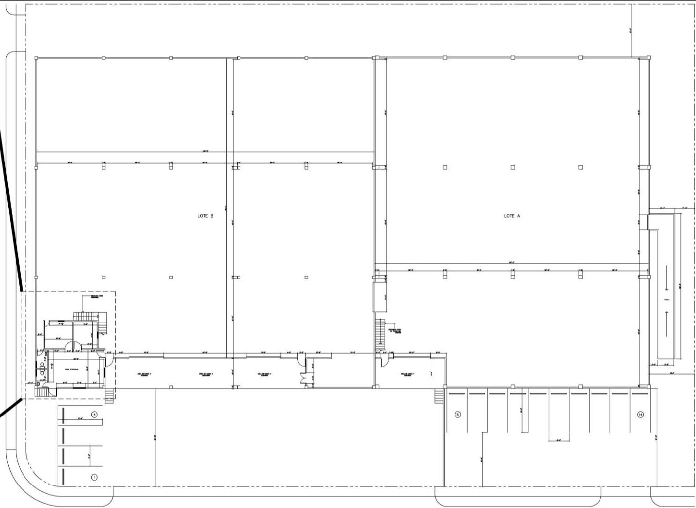
PLANTA DE PISO SCALE: 3/32"=1'-0"
